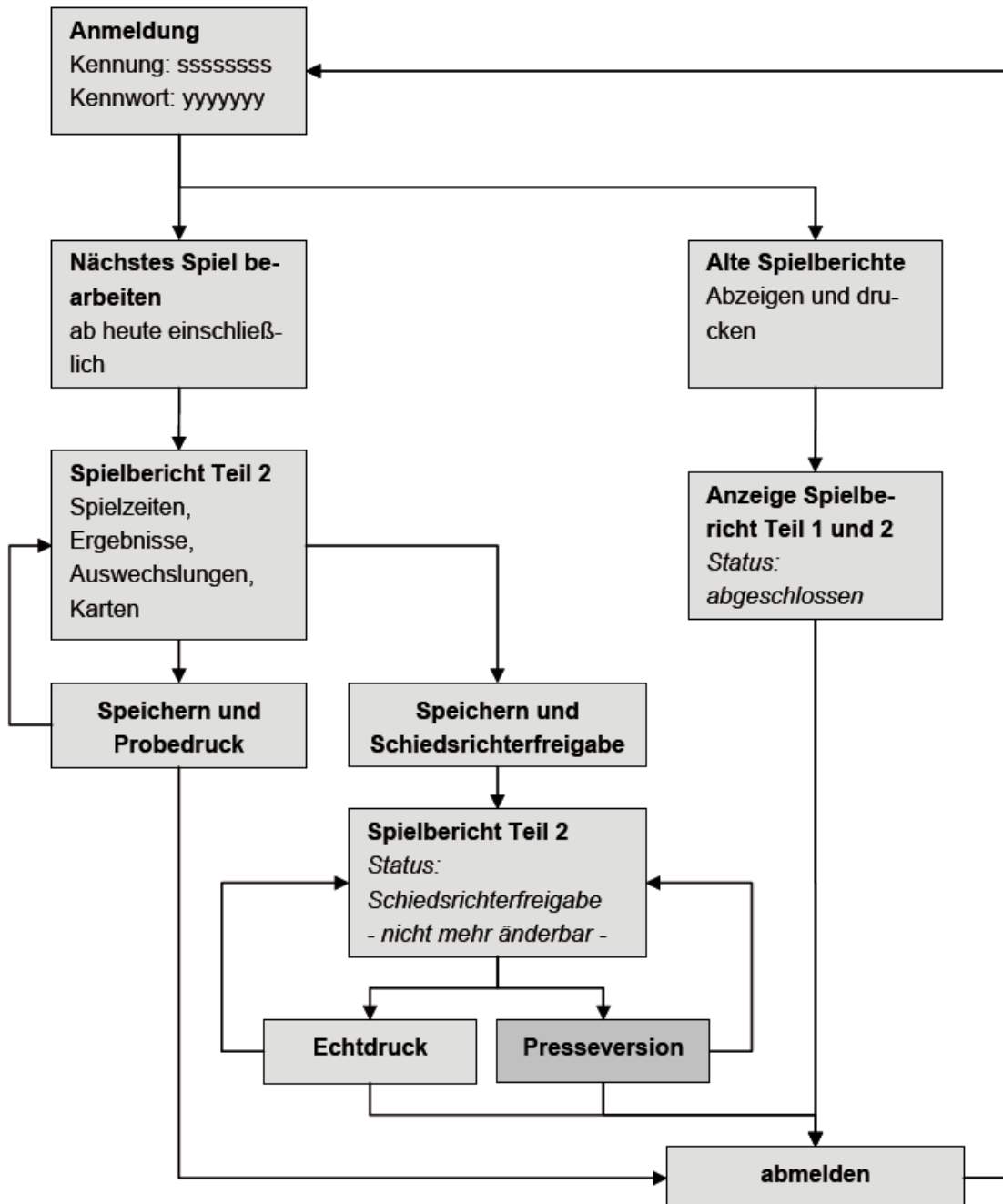
Abbildung 4: Dialogfluss der Anwendung bei der Rolle Schiedsrichter
